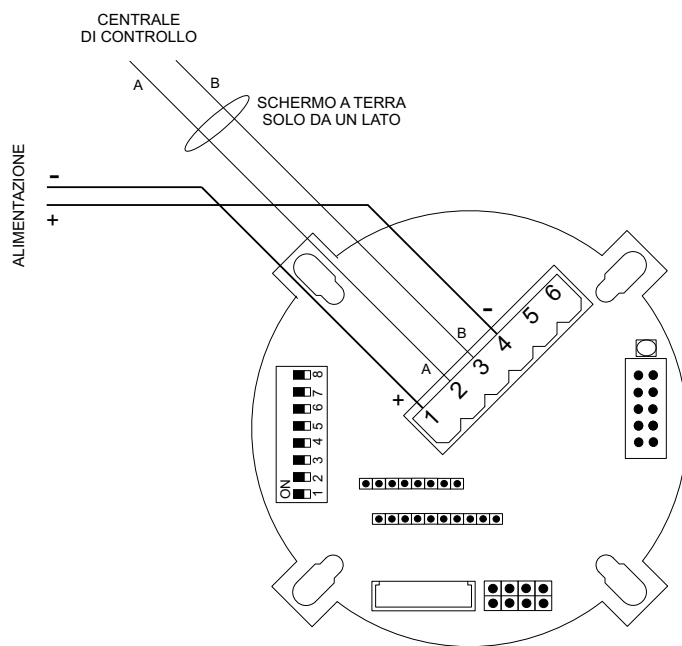
Figura 3) Collegamento rivelatore su bus seriale RS485
